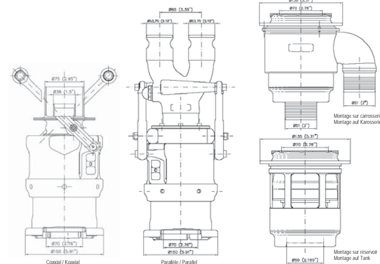
Dessin/Skizze 252-5 (Version B) (Accoupleur mâle / Kupplung männlich)
