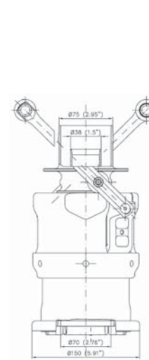
Dessin/Skizze 252-5 (Version B) (Accoupler mâle / Kupplung männlich)
