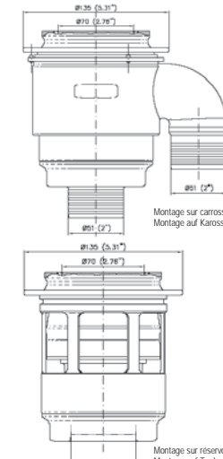
Montage sur réservoir Montage auf Tank
